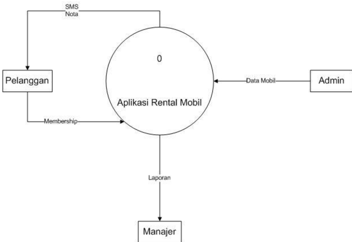
Diagram Konteks
